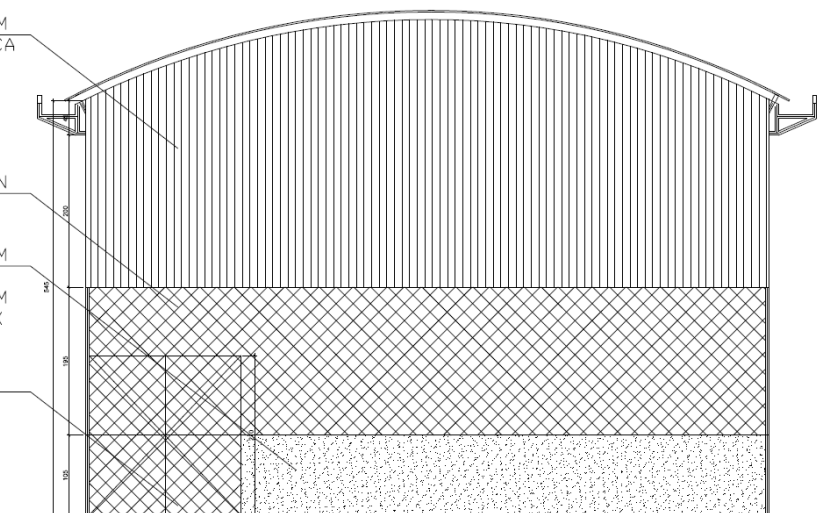
FACHADA PRINCIPAL ESC.: 1:50
